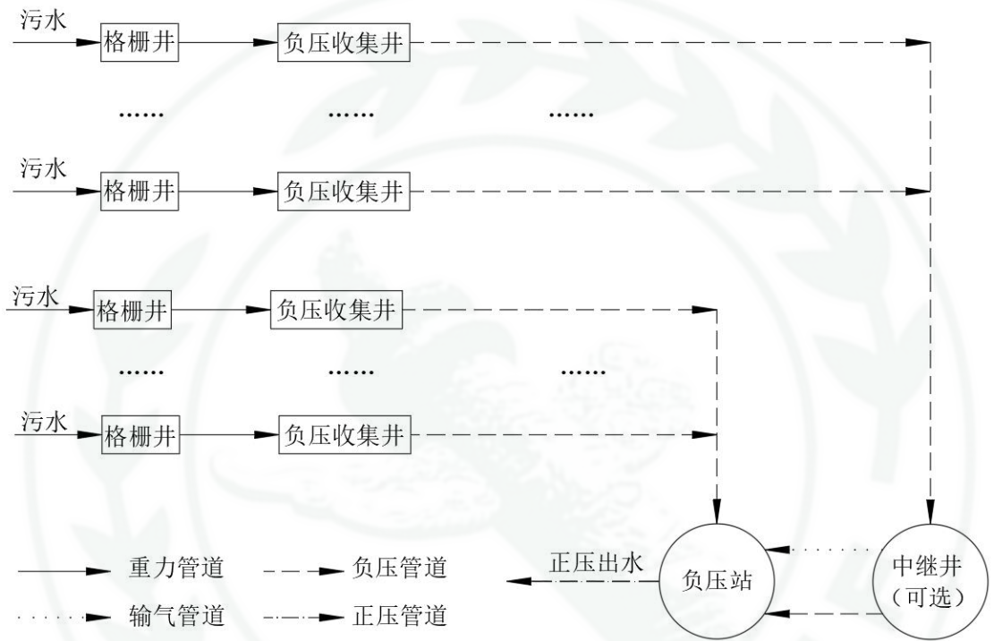
图 1 工艺流程图
